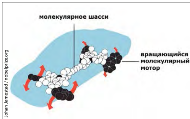
Модель молекулярной машины Феринги
