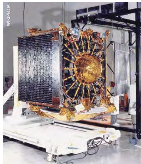
Спутник «Амос-1» перед запуском
